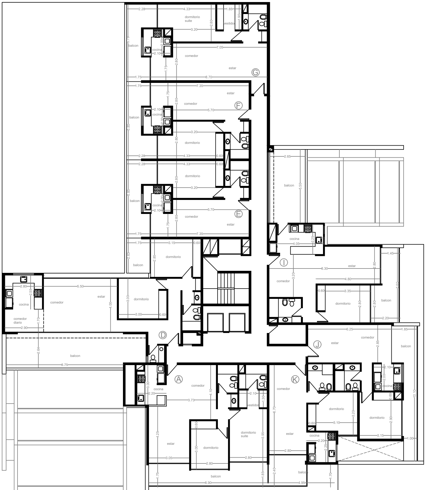
PLANTA PISO 7
