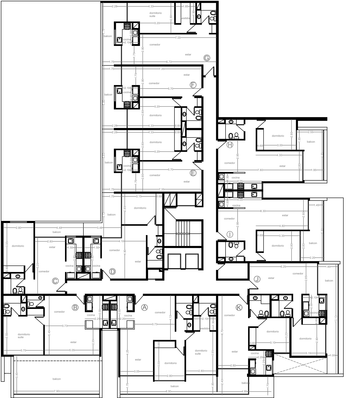
PLANTA PISO 4
