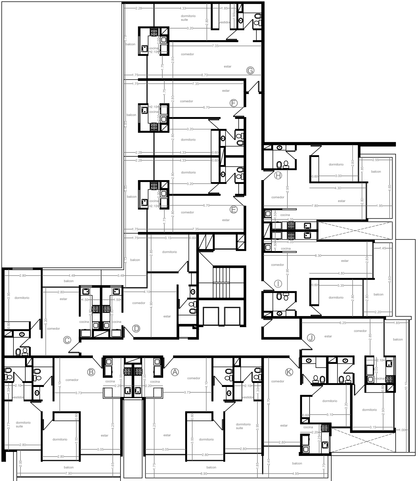
PLANTA PISO 1
