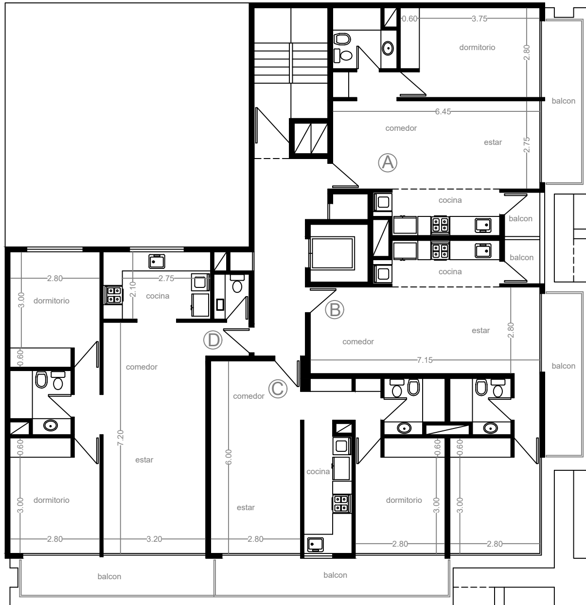
PLANTA PISO 7
