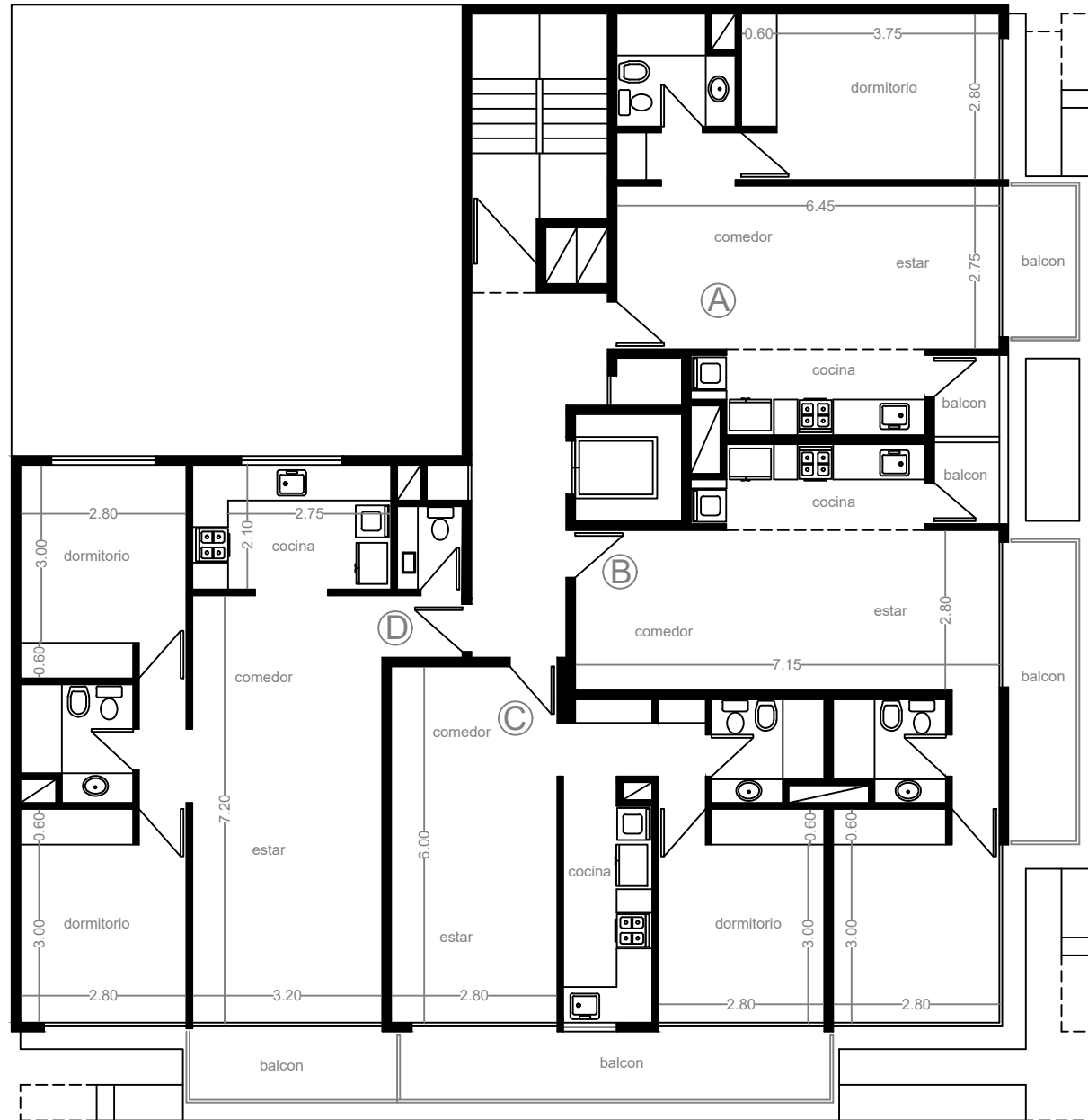
PLANTA PISO 6
