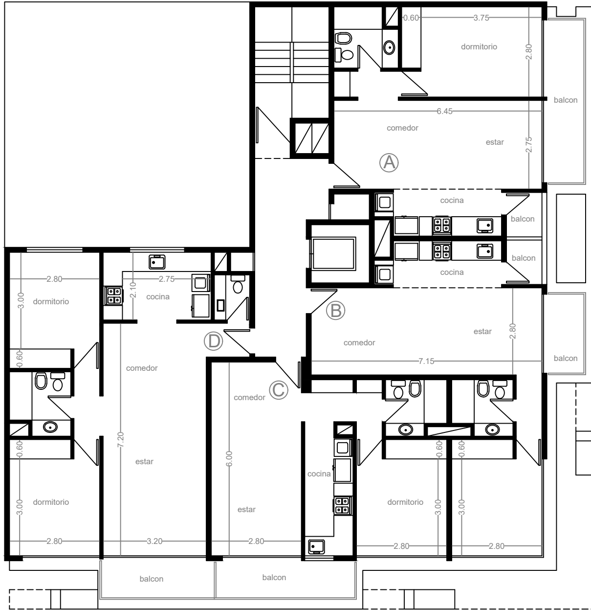
PLANTA PISO 4
