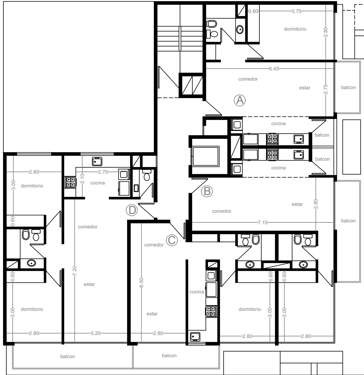
PLANTA PISO 3
