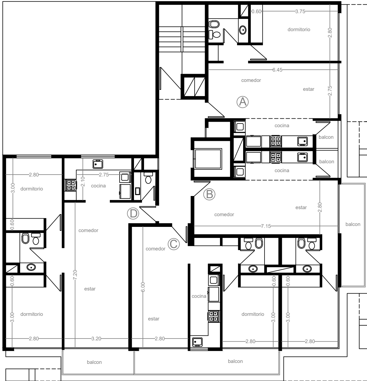
PLANTA PISO 1
