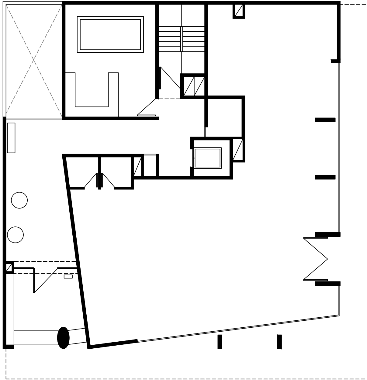
PLANTA PISO P.B.
