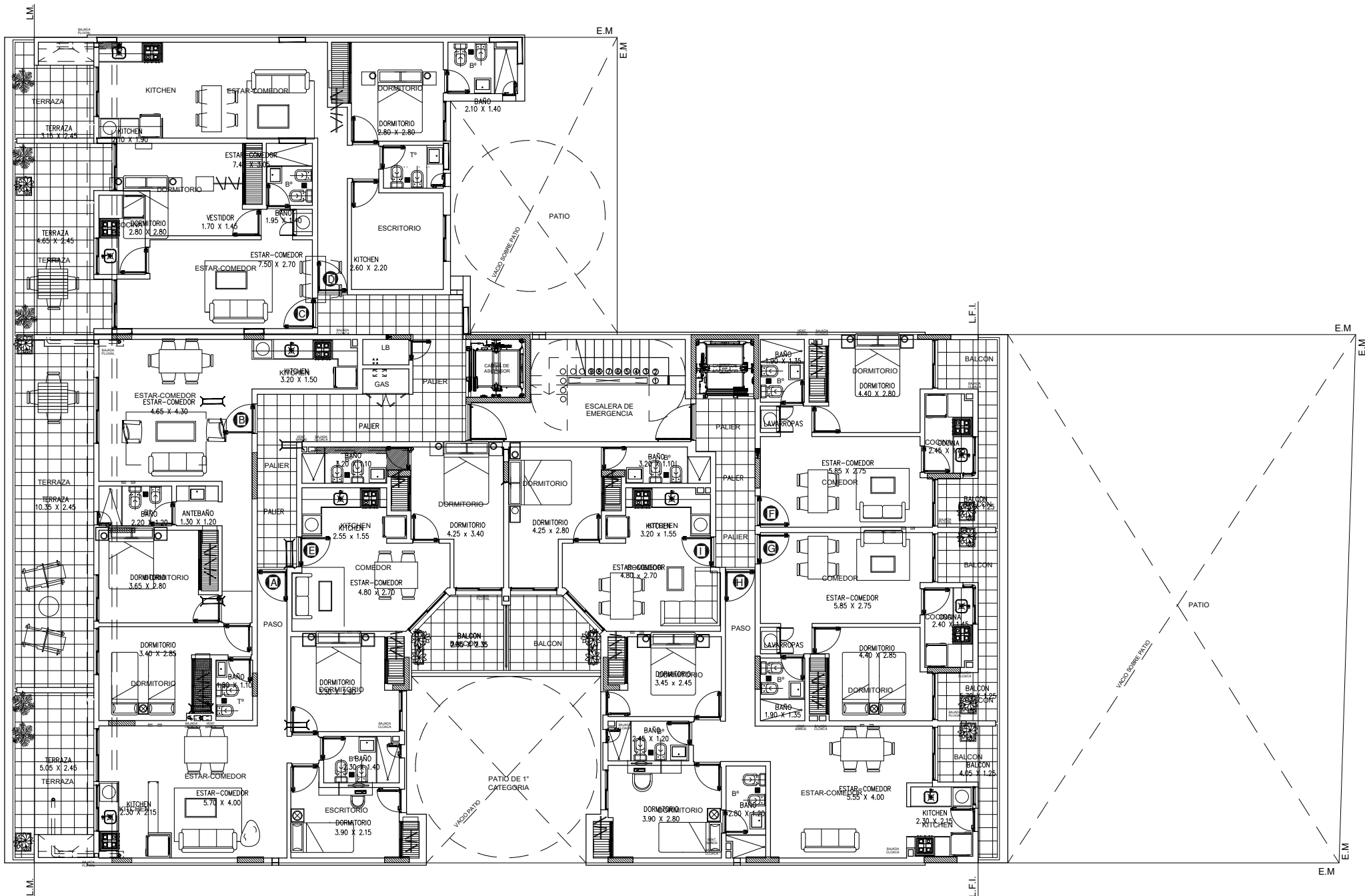
PLANTA 4° PISO
